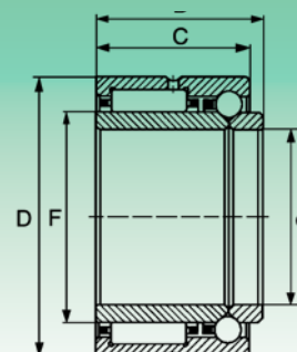
NKIB
