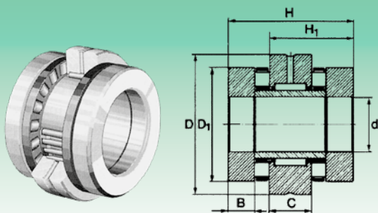
ZARN
