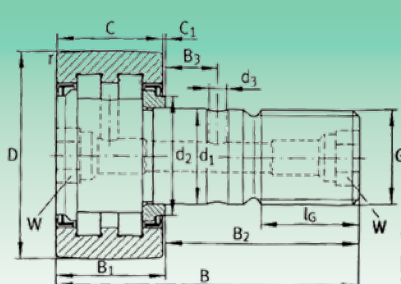
PWKR..-2RS
