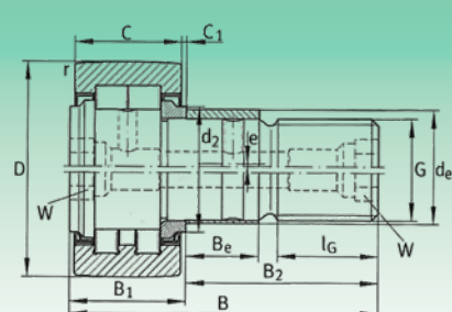
NUKRE PWKRE..-2RS
